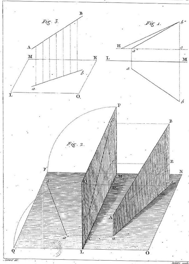
Figura 7 G. Monge, Planche I.
