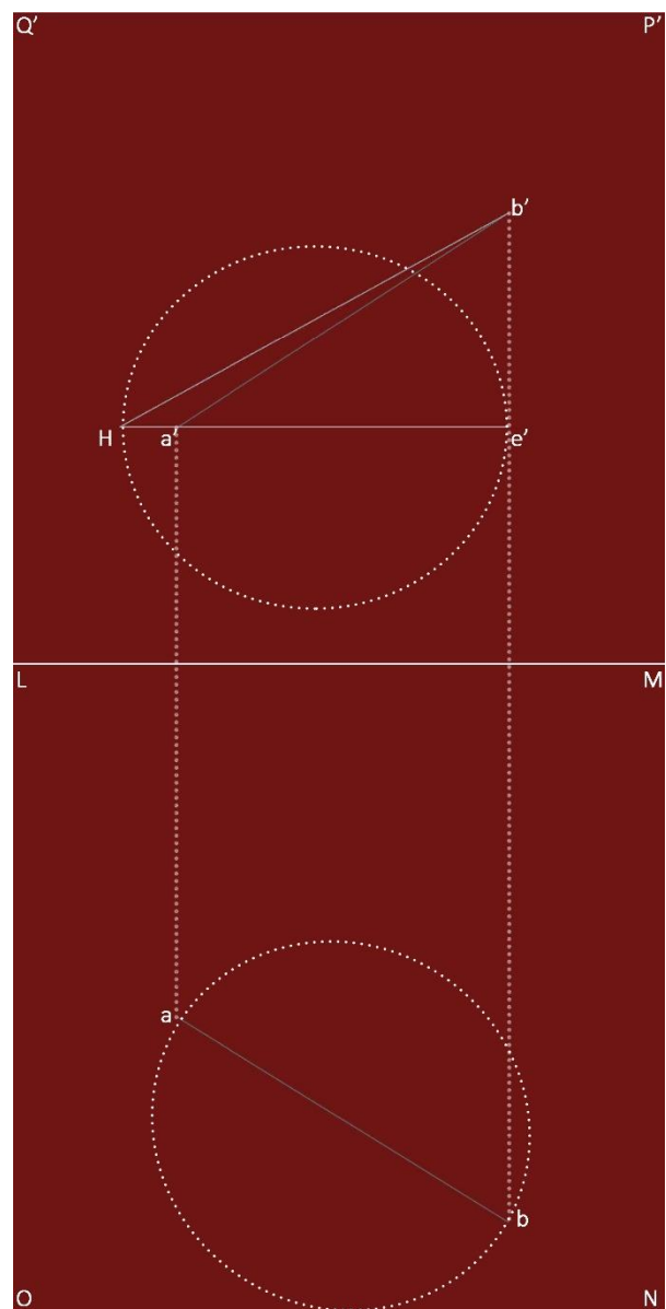
Figura 10 Digitalizzazione della Fig. 1 della planche I del trattato di Monge. Elaborazione grafica di I. Friso.
