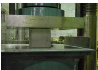
Calcestruzzo: prova di compressione diretta
