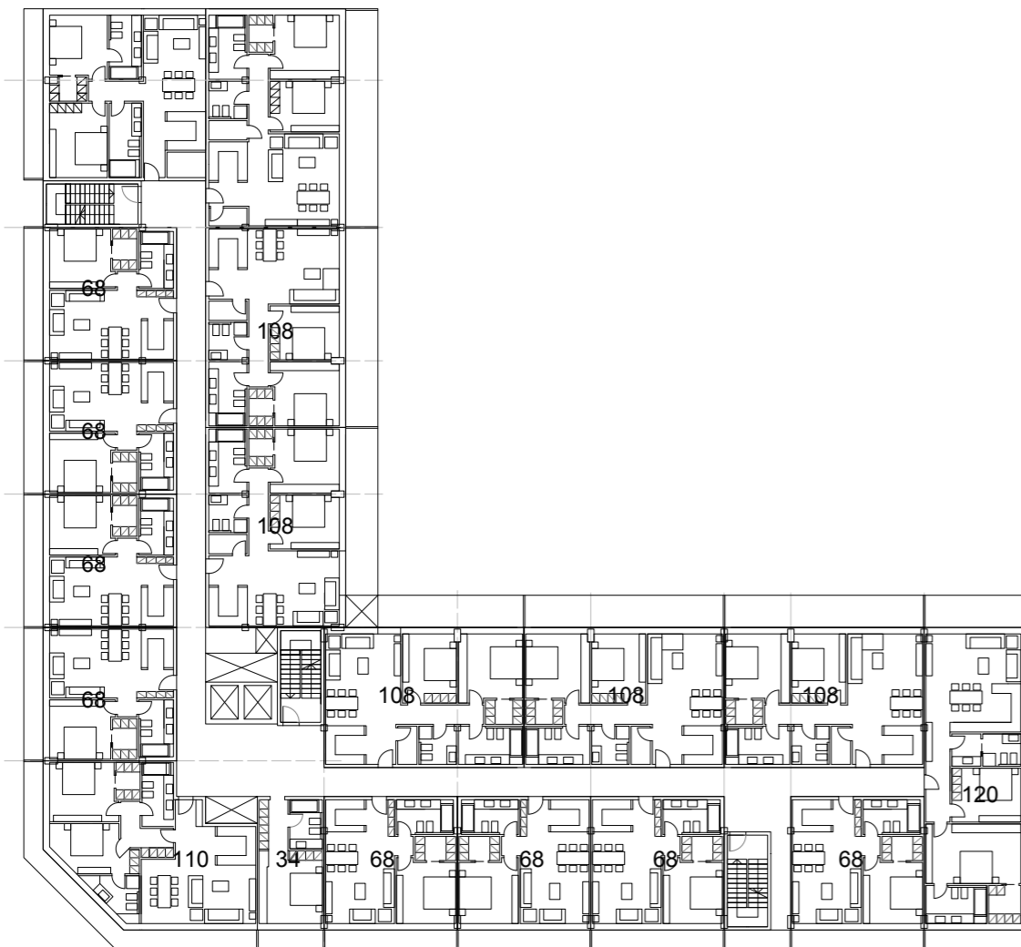
Piano tipo
