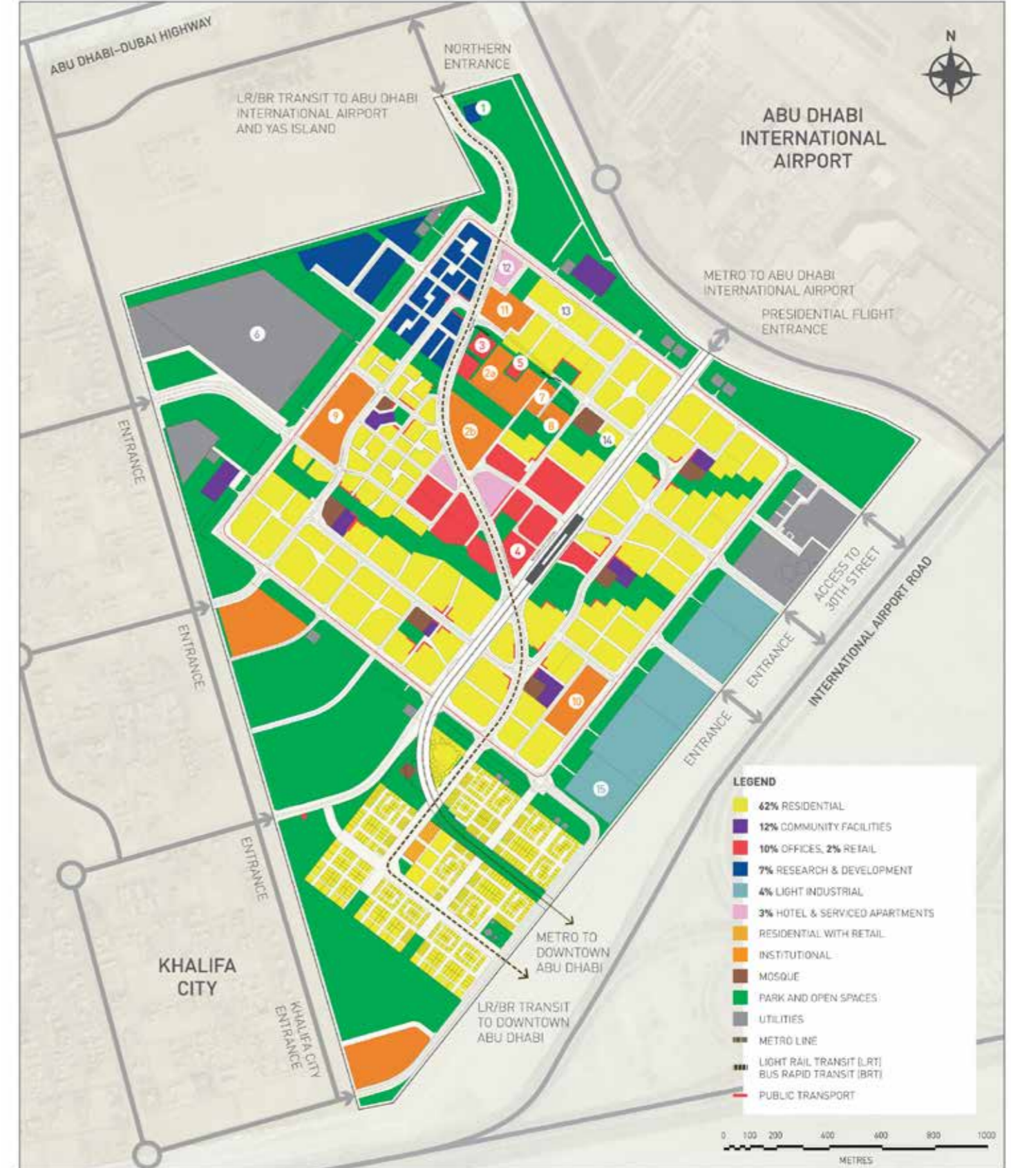
Sviluppo Masterplan
