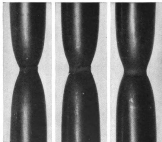
Barra di acciaio (Nadai 1950)
