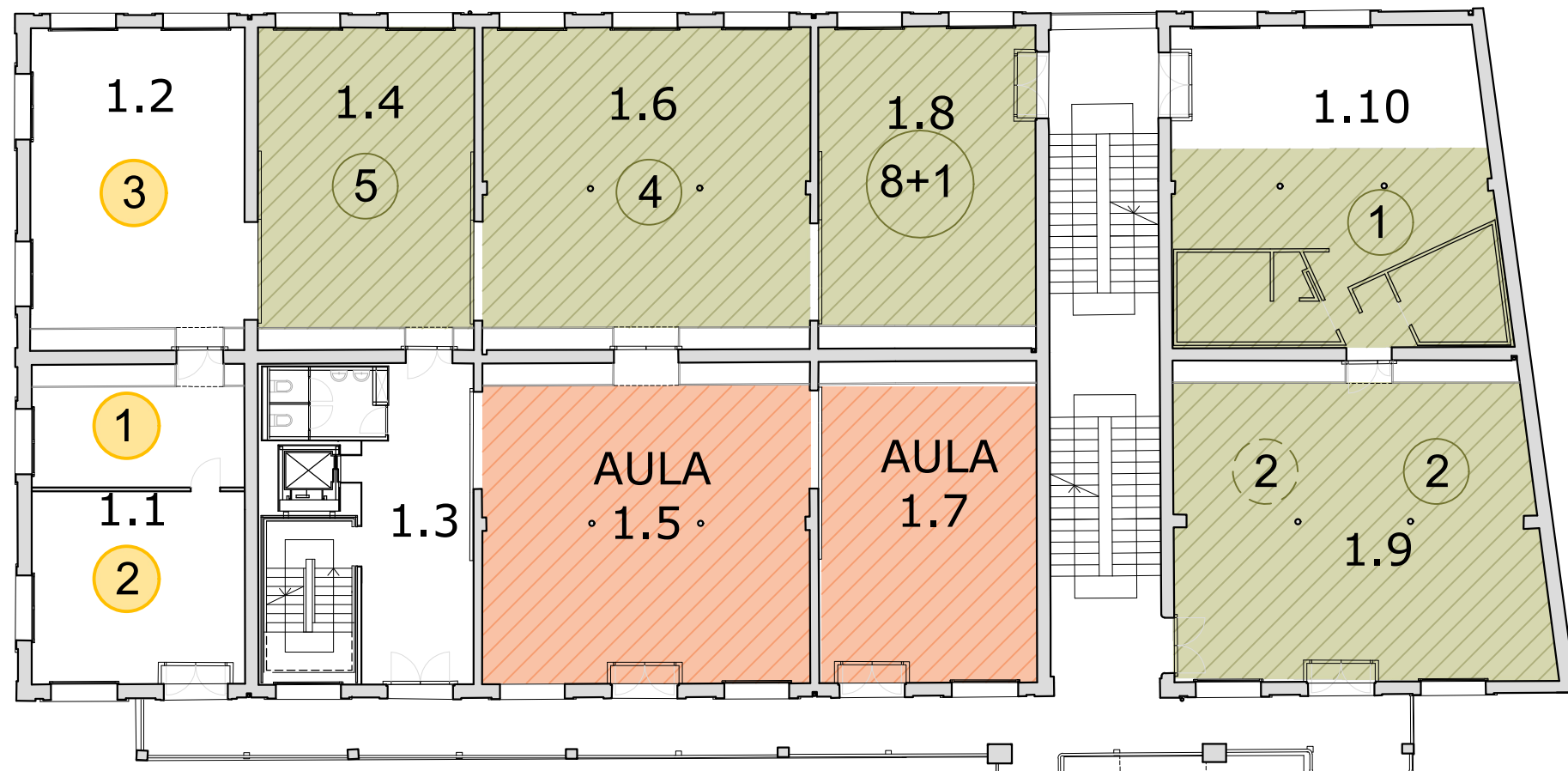
Magazzino 7 Primo Piano Scala 1:200
